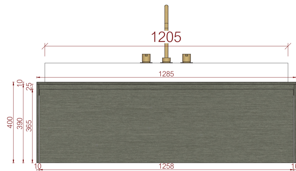
Vooraanzicht
