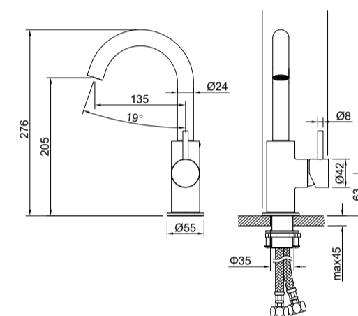
TTUV390111 Tuvalu wastafelmengkraan met draaibare uitloop bladmontage, zonder waste
