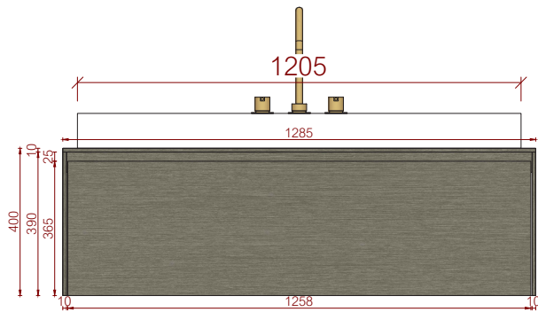
Vooraanzicht
